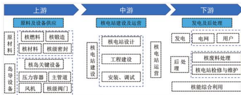
先进核能产业链示意图
